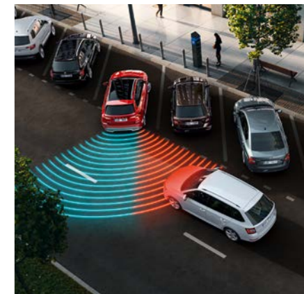
Rückfahrassistent Dieser Assistent, der zum Totwinkelassistenten «Blind Spot Detection» gehört und dieselben Radarsensoren nutzt, hilft Ihnen dabei, auch bei schlechter Sicht sicher rückwärts ausparkieren.
